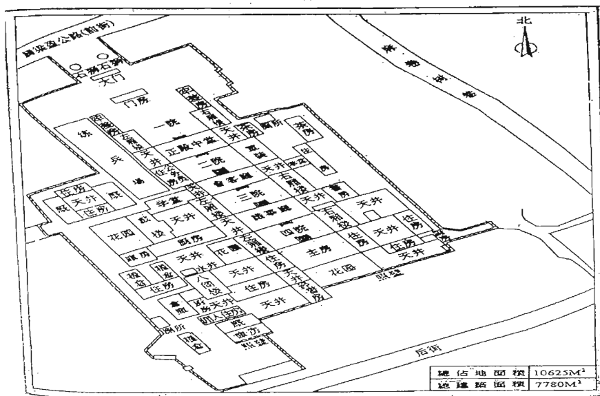
南甸宣撫司署平面圖
